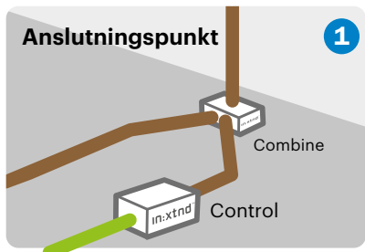
Inkoppling av In:xtnd™ Control och In:xtnd™ Combine
